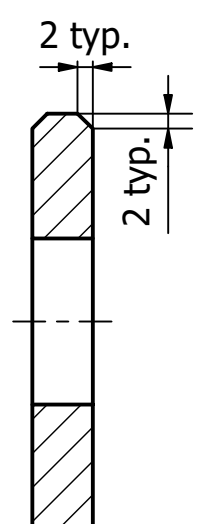
B-B ( 1 : 1 )
